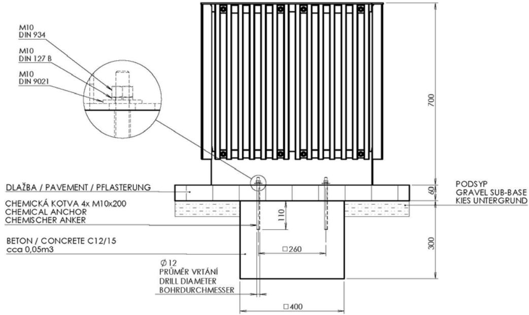
FL650 56.3kg
