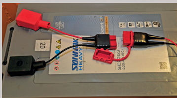
Hurtigkontakt sikrer mot feil kobling
