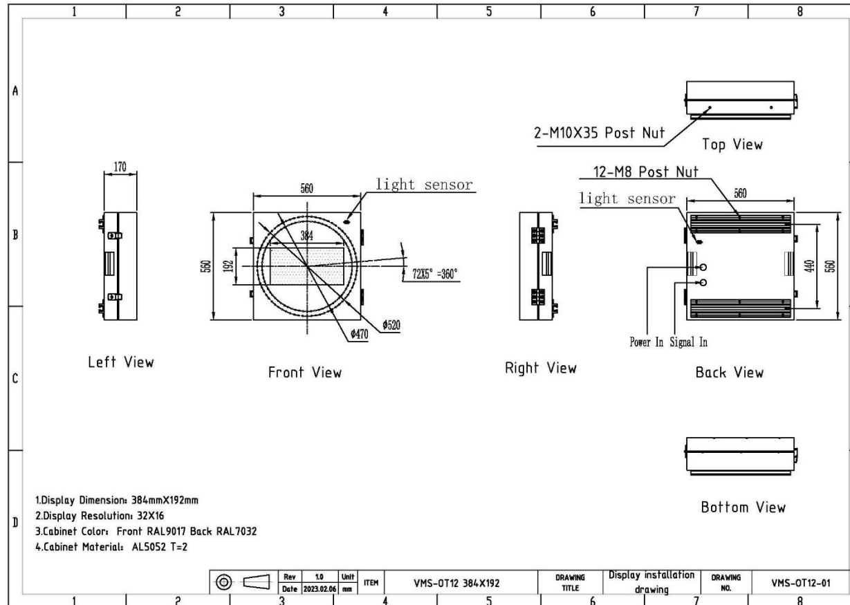
Figur 1: Sammenstillingstegning (GA)
