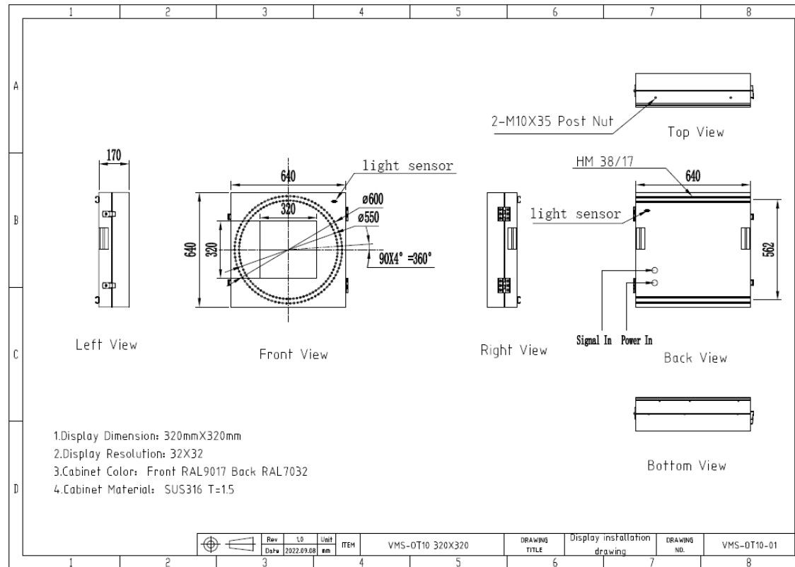
Figur 1: Sammenstillingstegning (GA)
