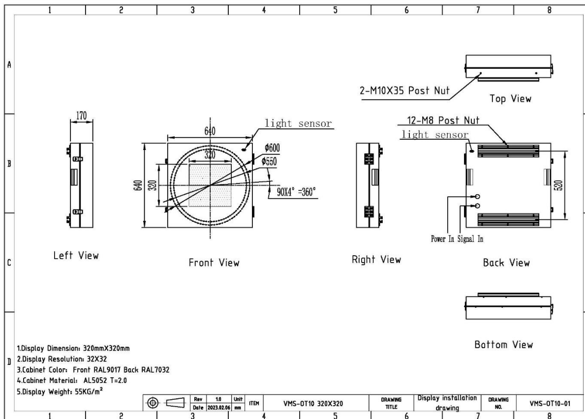
Figur 1: Sammenstillingstegning (GA)
