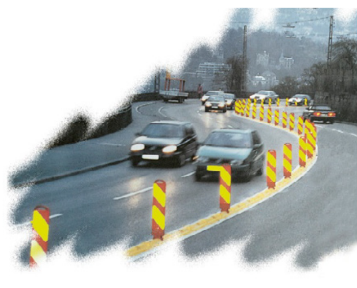
Klemmfix Hindermarkeringer montert på ledeskinne.
